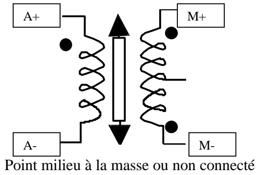
PONT COMPLET 4 ou 5 fils
